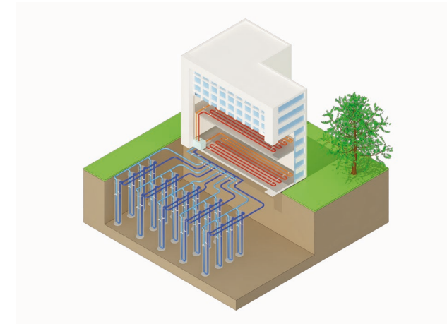
Champs de sondes géothermiques verticales ©ADEME-BRGM
