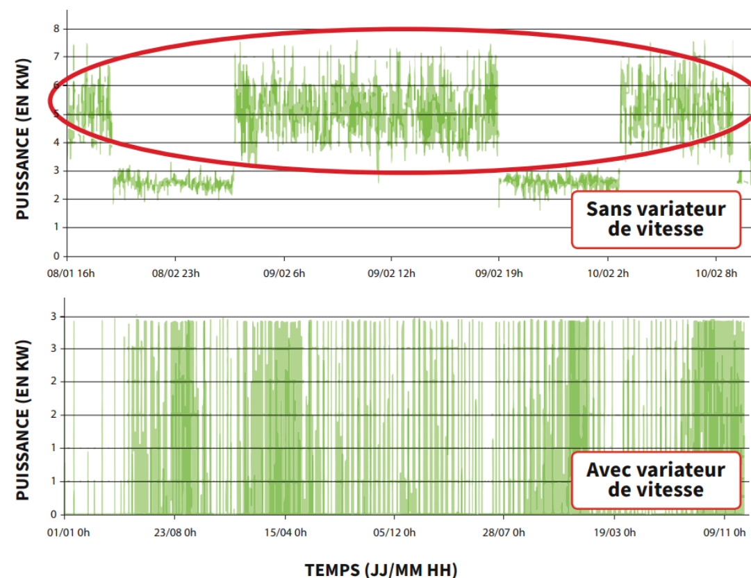
ÉVOLUTION DE LA PUISSANCE DE LA POMPE DE FORAGE
