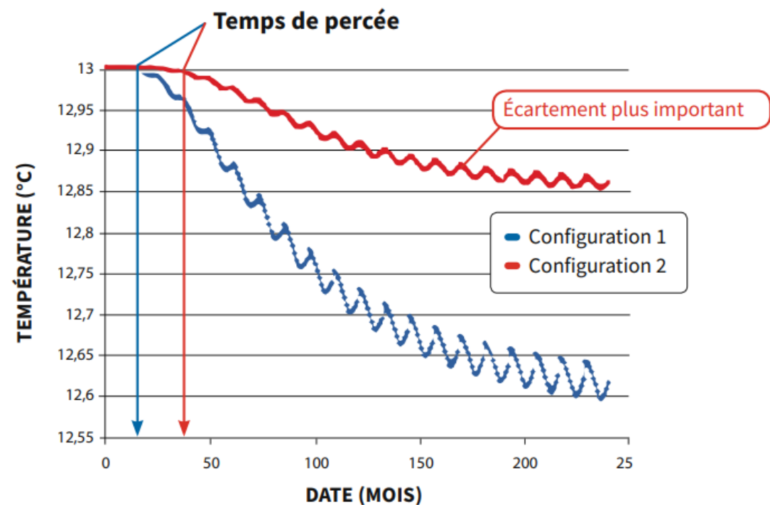
ÉVOLUTION DE LA TEMPÉRATURE AUX Puits DE PRODUCTION SELON DEUX CONFIGURATIONS D'ÉCARTEMENT Puits DE PRODUCTION - Puits D'INJECTION
