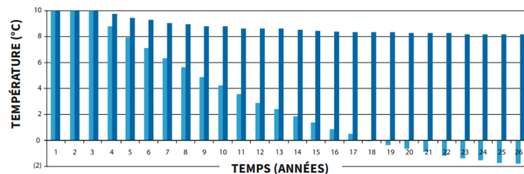
ÉVOLUTION DE LA TEMPÉRATURE DANS LE SOUS-SOL DANS LE CAS D'UN SOUS DIMENSIONNEMENT ET D'UN BON DIMENSIONNEMENT DU CHAMP DE SONDES
