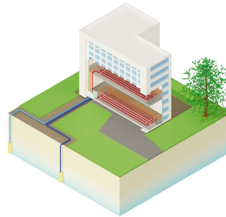
Captage sur nappe ©ADEME-BRGM
